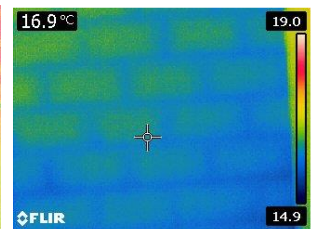
Figura 2.5 – Immagine termografica muro dall'esterno
