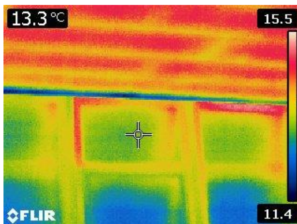
Figura 2.4 – Immagine termografica finestra
